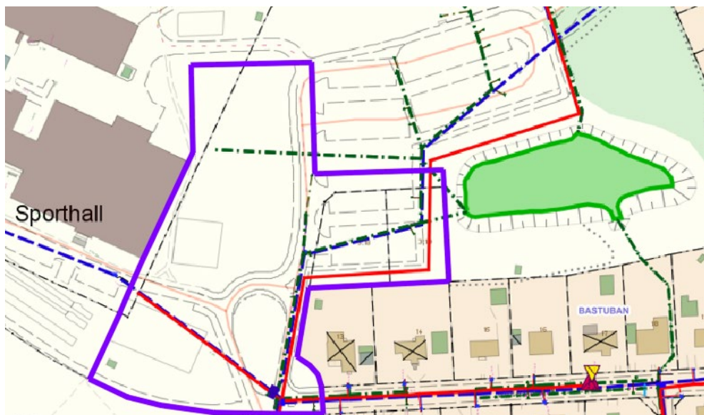
Figur 29: Kartan visar dagvattendammen öster om planområdet (den mörkgröna ytan i kartan) samt befintliga dagvattenledningar (med grönt streckade linjer) på fastighet Norrby 3:1 inom och utanför detaljplanensgränsen (markerad med lilafärgad kontur).
