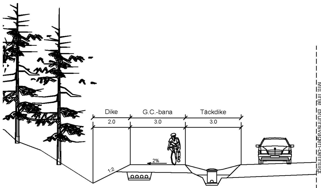
Figur 7: Skissen visar normal sektion med gång-och cykelbana längst Brunnsvägen.
