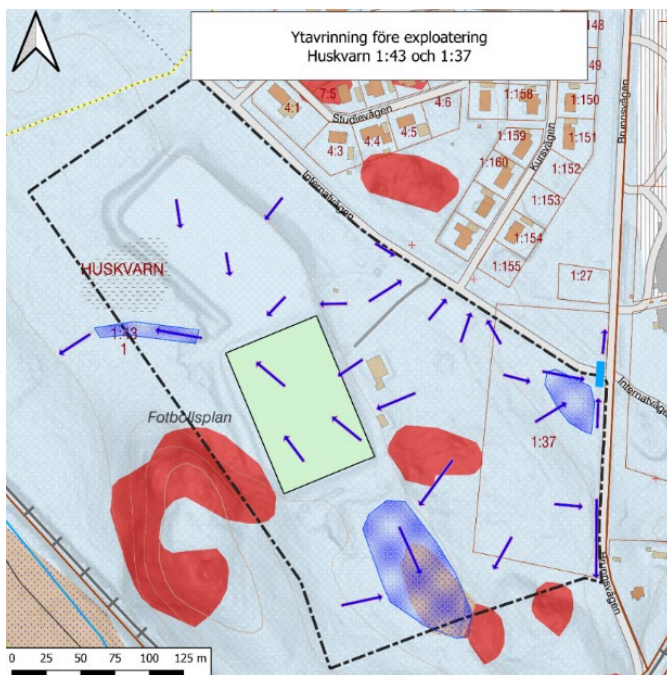
Figur 16: Illustration från dagvattenutredningen med bedömd ytavrinning och lokala lågpunkter. Kartan visar även befintlig vägtrumma under Internatvägen, markerad med turkos
